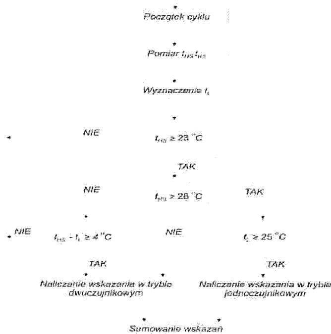
Rys. 2. Uproszczony schemat blokowy jednego cyklu pracy podzielnika elektronicznego
